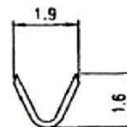
A-A SECTION
