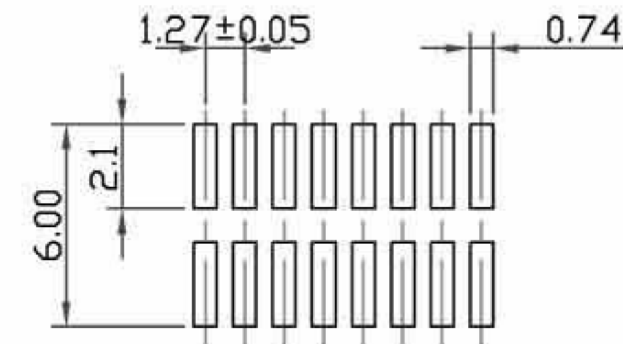
P.C.Board Layout
