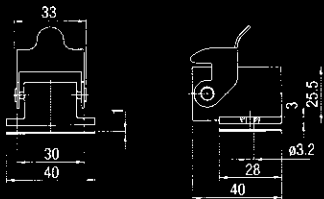
Montageausschnitt/Panel cut-out \varnothing 20
